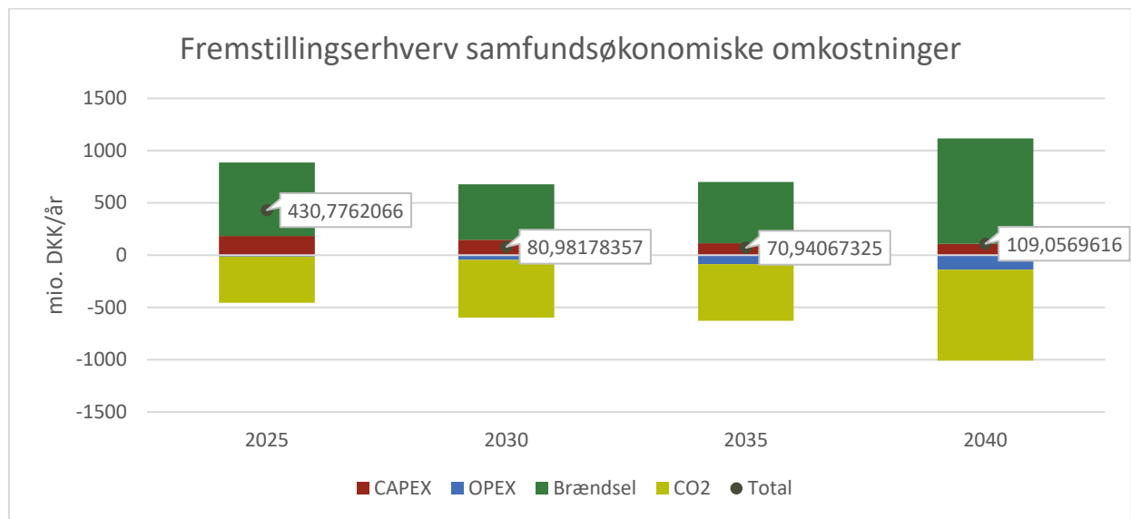
Figur 3-18 Samfundsøkonomiske meromkostninger af fremstillingserhverv i Transformationsscenarioet ift. referencen. Positive tal angiver en meromkostning
