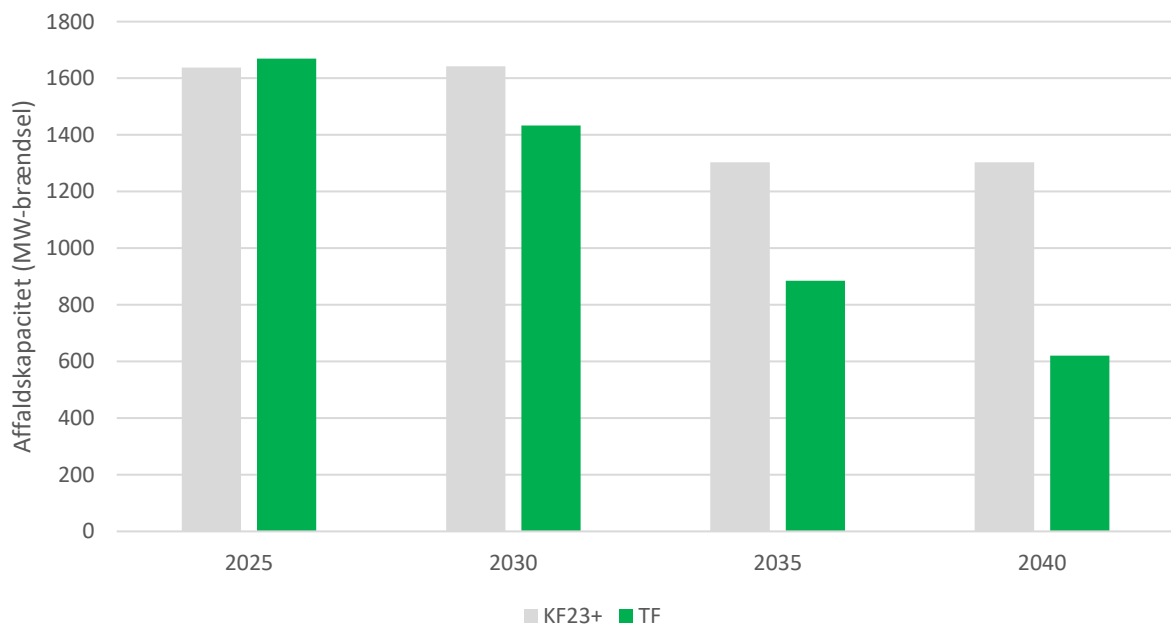
Figur 3-27: Indfyret kapacitet på affaldsværker i de opstillede scenarier
