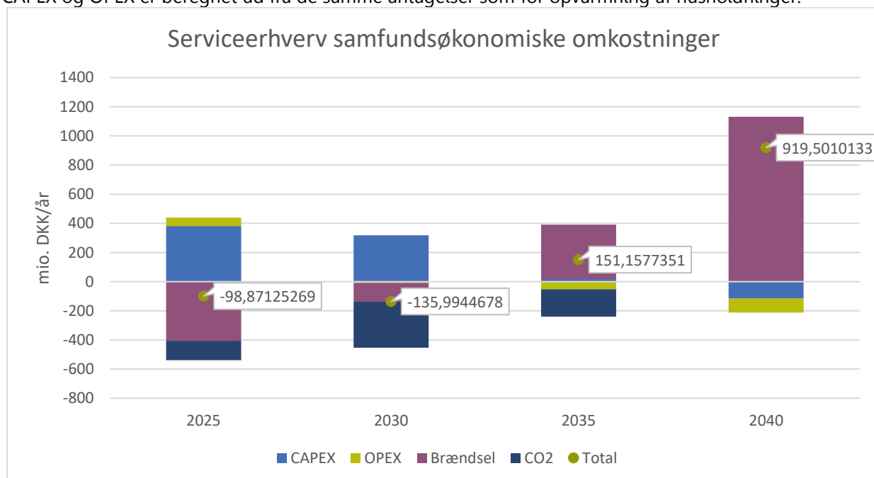
Figur 3-14 Samfundsøkonomiske meromkostninger af serviceerhverv i Transformationsscenarioet ift. referencen. Positive tal angiver meromkostninger
