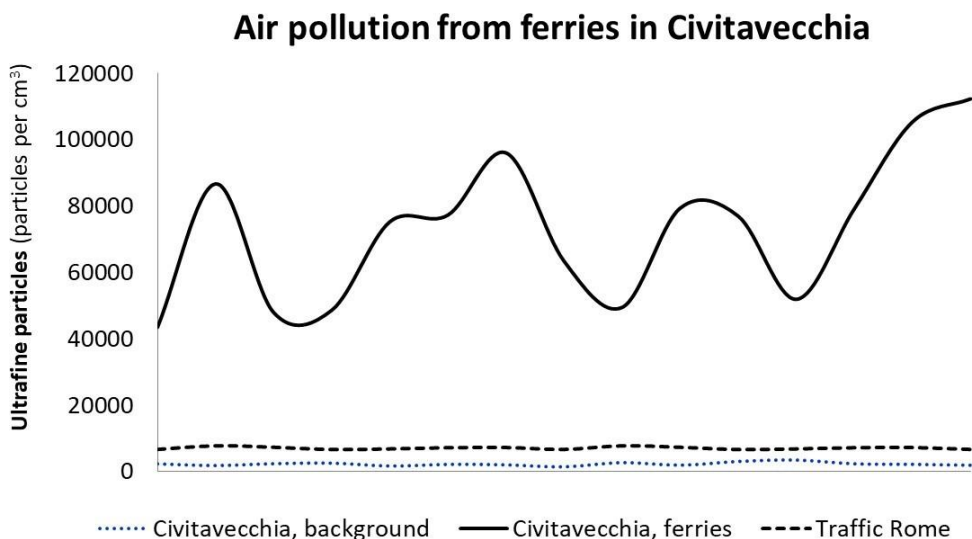
Figura 2: Misurazioni a Civitavecchia rispetto all'inquinamento da traffico nel centro di Roma
