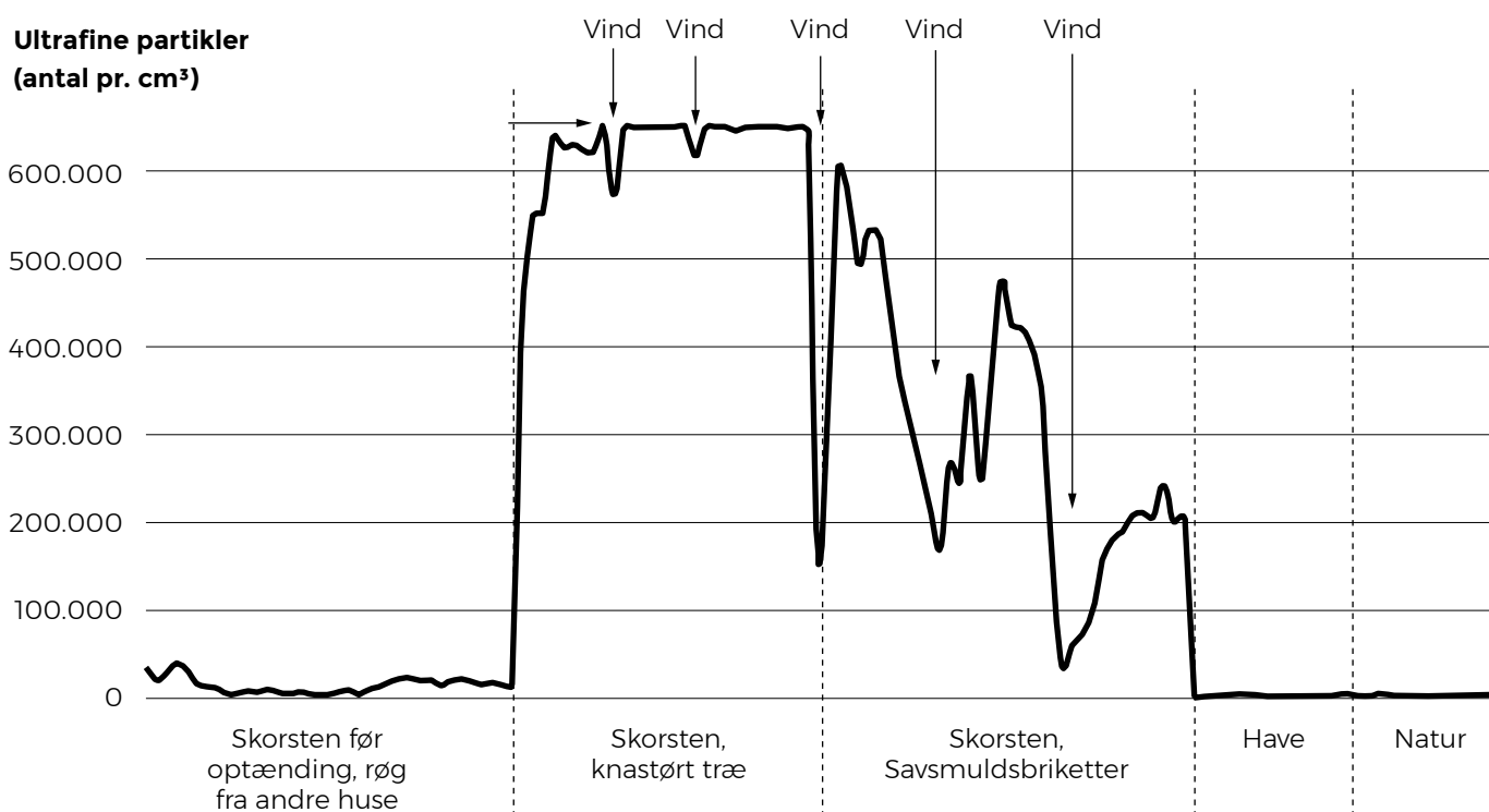
Figur 4: Måling af ultrafine partikler under optimale fyringsforhold.
